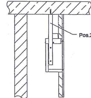
Deckenmontage
